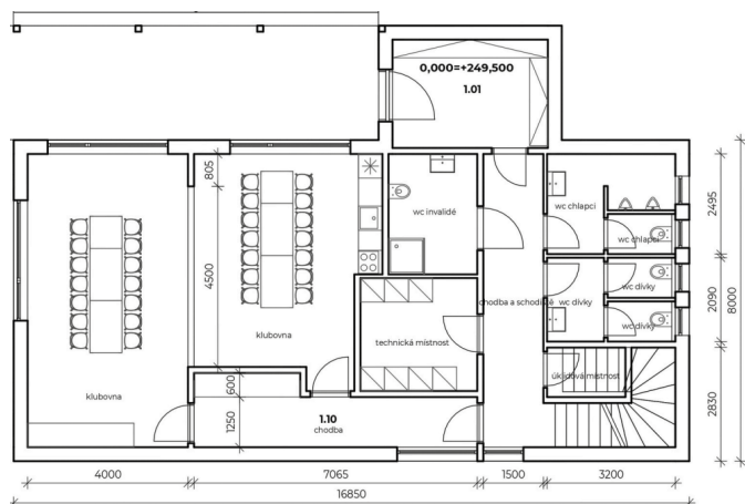
Půdorys přízemí klubovny
