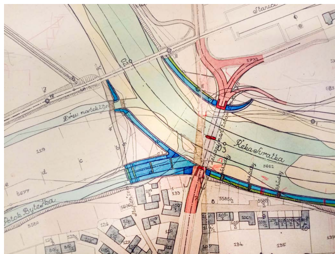
Plány nam úpravu břehů Svratky a nový betonový most Tišnovská
