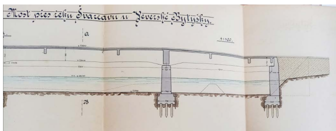
Jeden z návrhů plánů mostu
