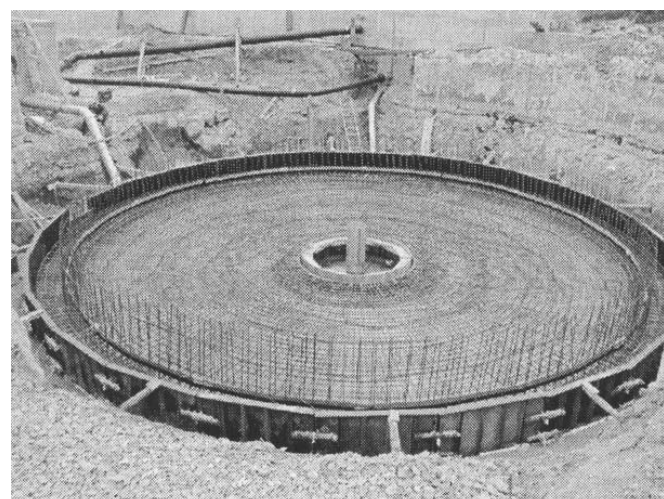
Dosazovací nádrž DN2
